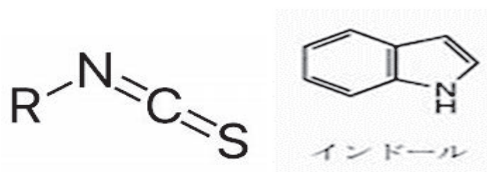
イソチオシアネートの基本骨格
