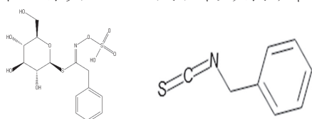
グルコトロペオリン ベンジルイソチオシアネート
